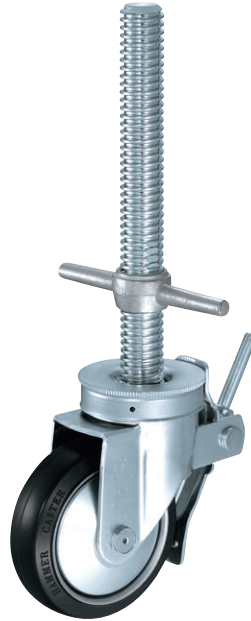
515SA-RB 150mm (仮設工業会認定キャスター)
