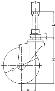
420 2EU-R 75mm(三ツ又形状)
